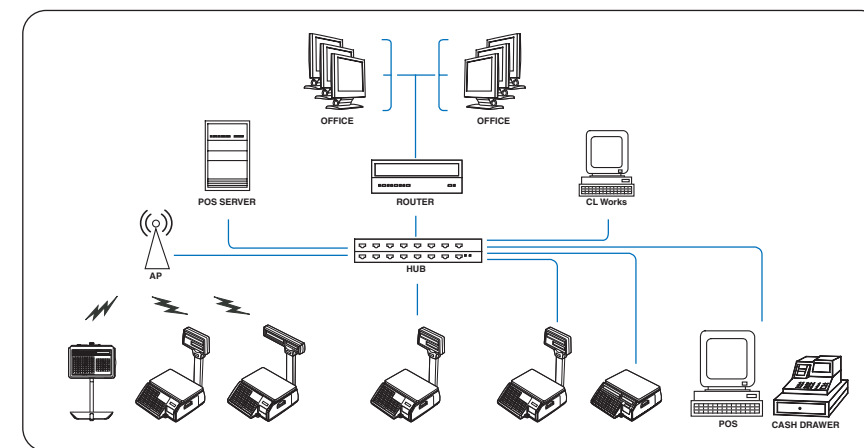
Kabelgebundener / WLAN-Verbund
